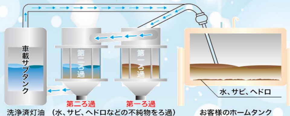
ホームタンク洗淨の流れ
